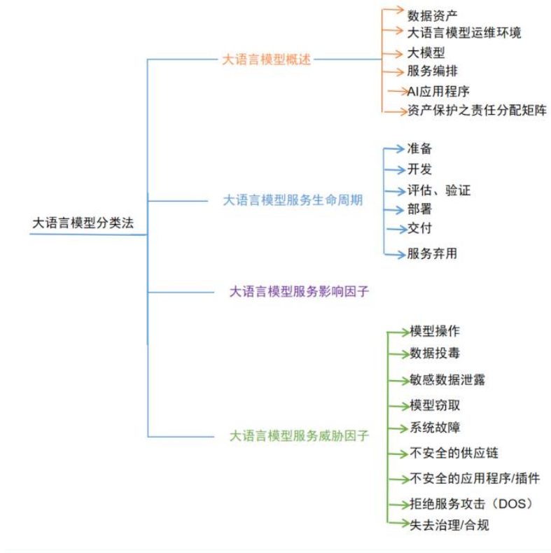
图 1: CSA LLM 威胁分类法
